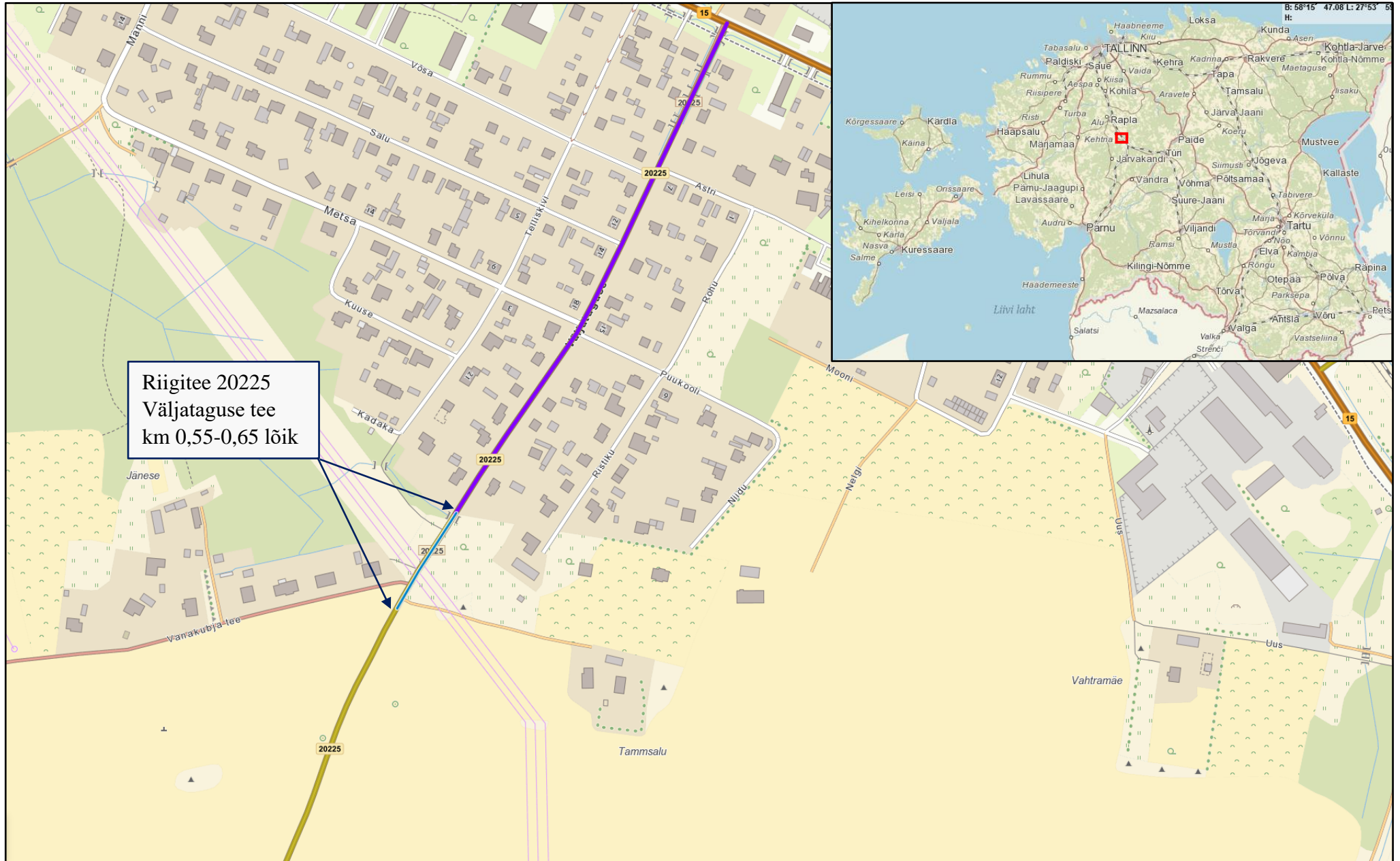
Lisa. Projekteeritava riigitee 20225 Väljataguse tee km 0,55-0,65 asuva teelõigu asukohaskeem
